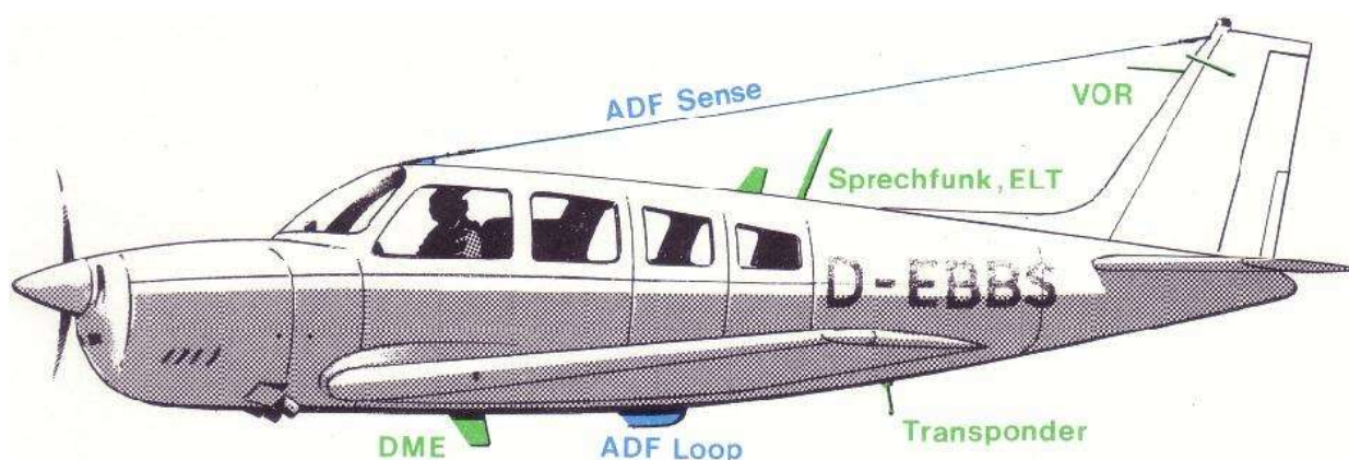
Abb. 4: Antennen an einem Flugzeug
