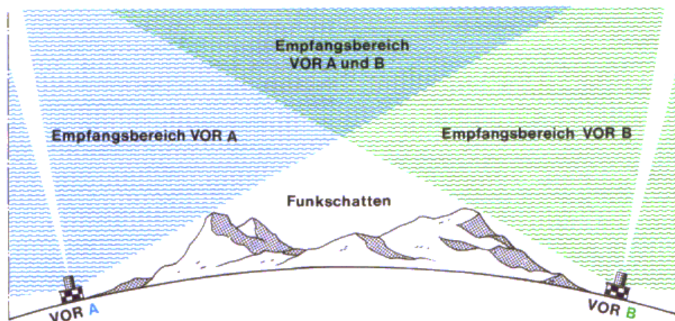
Abb. 3: Empfangsbereich der VHF-Sender (Schnitt durch die VOR-Ausstrahlung)
