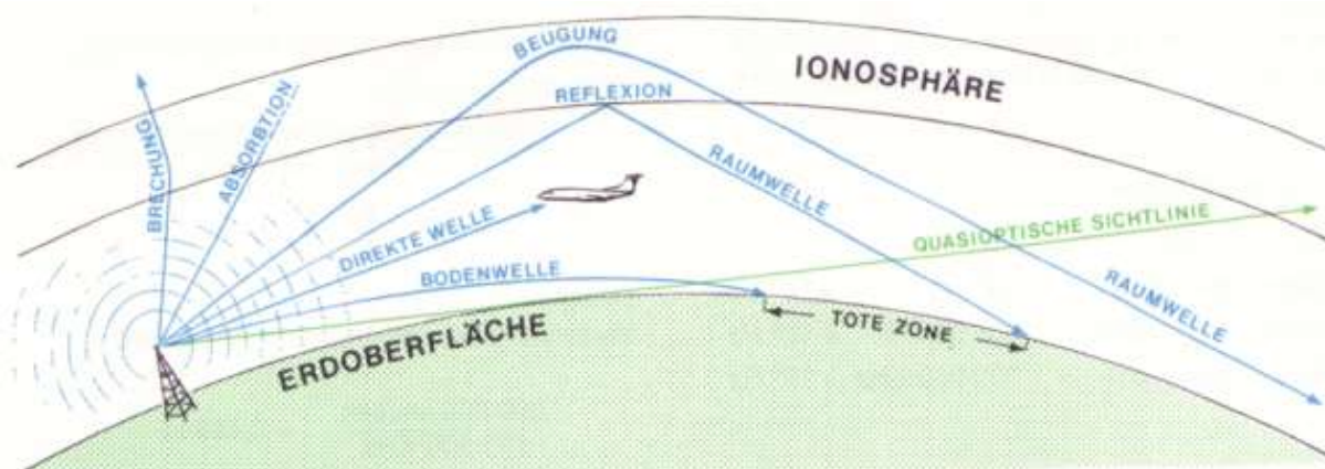
Abb. 2: Ausbreitung der Funkwellen
